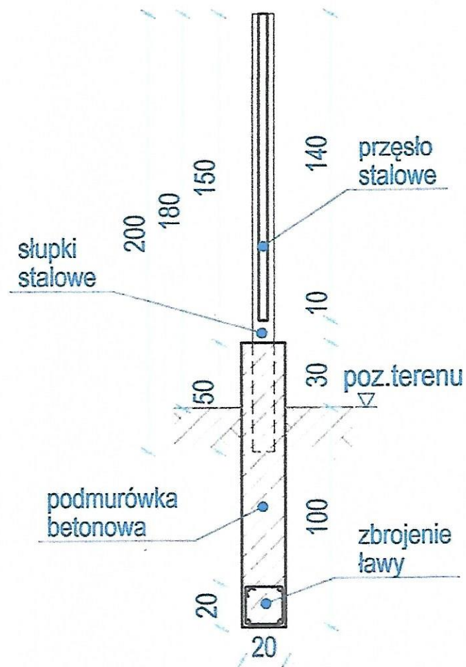
Przekrój przez projektowane ogrodzenie
